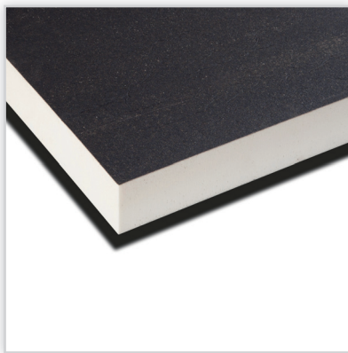
EUROTHANE BI-4/BI-4A. Bezfreonowa, twarda poliuretanowa płyta termoizolacyjna, pokryta obustronnie bitumizowanym włóknem szklanym. Zastosowanie: Bi-4 – na płaskich dachach i tarasach pod hydroizolacyjną membranę bitumiczną, alternatywa dla styropapy; Bi-4A – na podłożu betonowym pod klejoną membranę, w przypadku konieczności wyrobienia spadku. \lambda_d [W/(mK)]: 0,026. Wymiary [mm]: 1200/600/(30-120).
