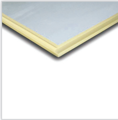
EUROWALL 21. Bezfreonowa płyta izolacyjna z rdzeniem z twardej pianki PIR w okładzinie z szarego laminatu paraizolacyjnego (papier typu kraft+folia aluminiowa), gdzie jedna strona jest matowa, a druga odblaskowa – skierowana na zewnątrz budynku. Wykończenie: obróbka standardowa na pióro-wpust. Zastosowanie: mury szczelinowe, ściany trójwarstwowe. \lambda_d [W/(mK)]: 0,021. Wymiary [mm]: 1200/600/(30-120).
