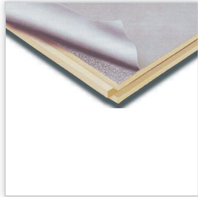
POWERROOF. Bezfreonowa, termoizolacyjna płyta z rdzeniem z pianki PIR, obustronnie karbowana folią aluminiową (na wierzchu dodatkowo wodoodporna folia RECTIVENT). Wykończenie: dookoła na pióro-wpust. Zastosowanie: termoizolacja nakrętkowa dachów skośnych. Zalety: jednolita izolacja bez mostków termicznych, szybki montaż nawet przy różnym rozstawie krokwi, renowacja bez wymiany wykończenia poddasza. \lambda_d [W/(mK)]: 0,022. Wymiary [mm]: 1200/2500/(60, 80, 100, 120, 140, 160, 180).
