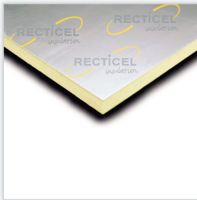
EUROTHANE SILVER. Twarda płyta PIR wykonana z pianki poliizocjanurowej (TAUfoam by Recticel) pokryta wielowarstwowym laminatem odpornym na przenikanie gazów, zawierającym w swojej strukturze aluminium. Zastosowanie: termoizolacja dachów płaskich na podłożu z blachy trapezowej stosowana pod mocowaną mechanicznie jednowarstwową syntetyczną hydroizolacją lub dwuwarstwowo pokrycie bitumiczne. \lambda_d [W/(mK)]: 0,022. Wymiary [mm]: (600, 2500)/1200/(30-150).
