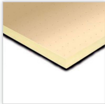
POWERDECK F. Bezfreonowa, twarda poliizocjanurowa płyta termoizolacyjna, obustronnie pokryte okładziną w włókna szklanego. Zastosowanie: termoizolacja dachów płaskich pokrytych membraną wodoodporną. Przyklejona ciepłym lub zimnym bitumem, jako element termoizolacji w układzie B50, zgodnie z zaleceniami dostawcy systemu. \lambda_d [W/(mK)]: 0,026. Wymiary [mm]: 1200/600/(30-140).
