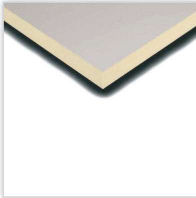
EUROFLOOR 300. Bezfreonowa, twarda, poliuretanowa płyta termoizolacyjna w okładzinie z laminatu typu kraft aluminium odpornego na korozję alkaliczną. Zastosowanie: izolacja posadzek, również pod ogrzewanie podłogowe. \lambda_d [W/(mK)]: 0,024. Wymiary [mm]: 1200/2500/(20-120). Odporność na nacisk podwyższona do 300 kPa.
